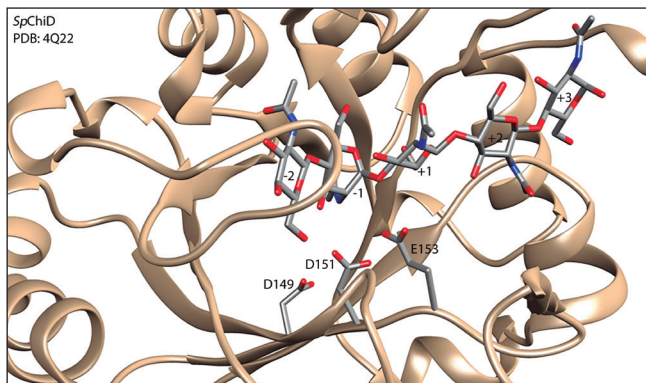
FIGURA 3. Centre actiu de la quitinasa SpChiD (PDB: 4Q22). Model del complex amb DP5 per docking .
